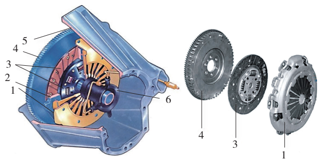
图 1-1-3 单片离合器
