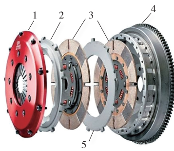
图 1-1-4 双片离合器
