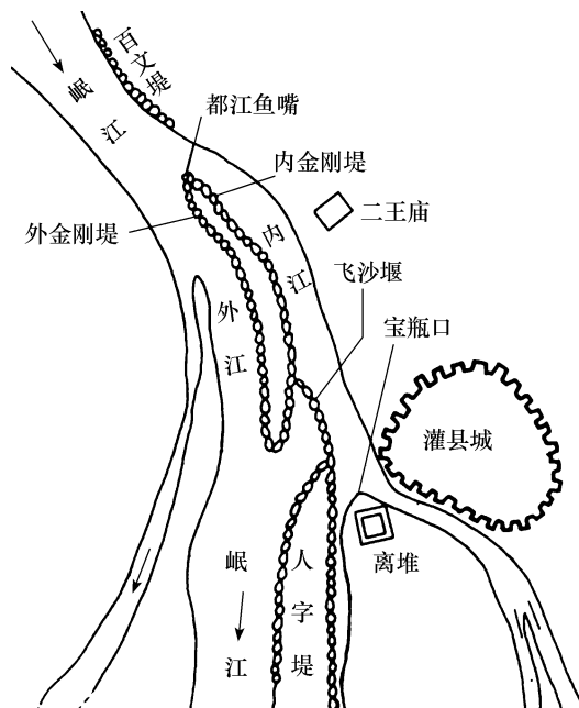
图 1-9 都江堰
