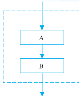
图 1-13 顺序结构
