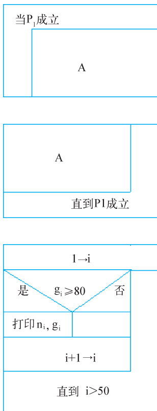
图 1-18 循环结构
