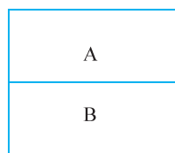
图 1-16 顺序结构
