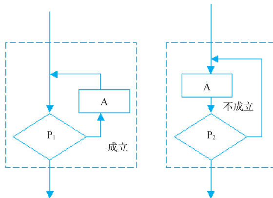
图 1-15-1 循环结构-1
