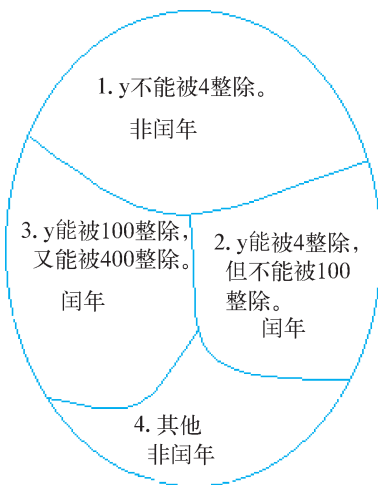
图 1-8 闰年判断
