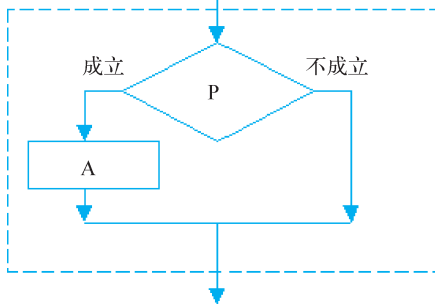
图 1-14 选择结构
