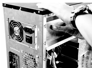
图 1-22 机箱电源安装
